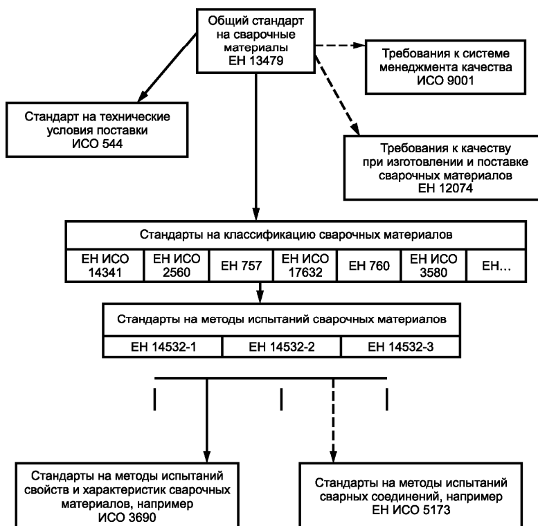
Рисунок 1 — Структурная схема взаимодействия документов, приведенных в настоящем стандарте
