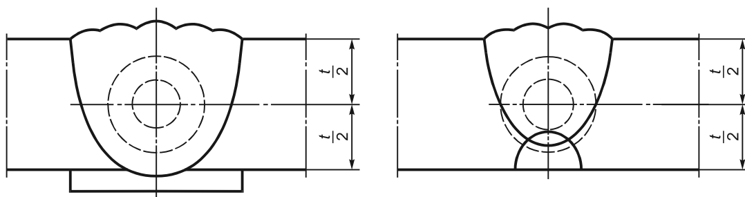
а) Контрольный образец для испытания металла шва по ЕН 1597-1
