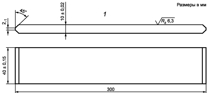
Рисунок 5 — Размеры контрольного образца для испытания на сопротивляемость образованию трещин программируемым деформированием (PVR-test)
