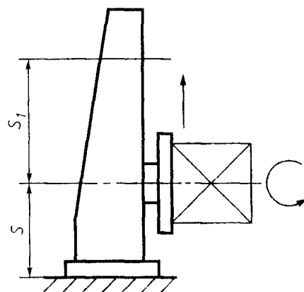
Рисунок А.2 — Кантователь центровой с подъемными центрами
